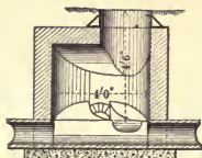
FIG. 3. SHALLOW MANHOLE.
